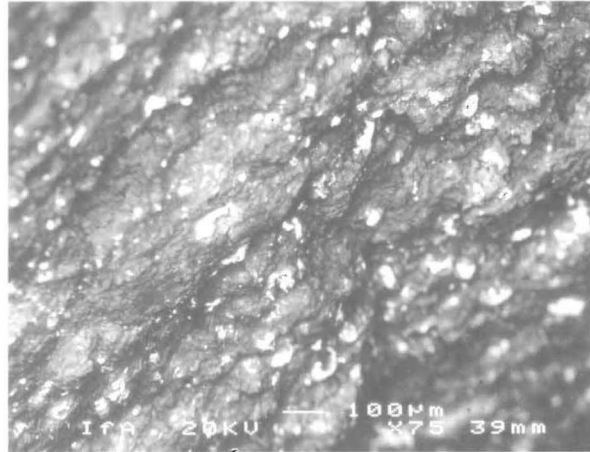
Abb. 4: RE-Aufnahme eines Teils der Innenwand aus Abb. 3. Die Metallspuren erscheinen hell auf der dunkleren Keramik. Die tropfen- bis fetzenförmigen Spuren erreichen Größen zwischen 10 und 100 µm.
