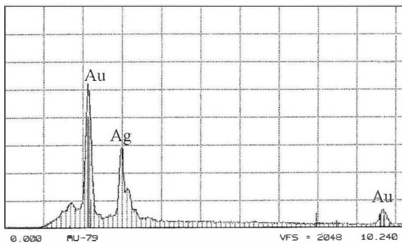
Abb. 5: EDX-Spektrum eines besonders silberreichen Metallpartikels. Der höchste Peak (links bei 2,2 KeV) ist die M-Linie von Gold, der nächsthöhere Peak (links der Mitte bei 3 KeV) ist die L-Reihe von Silber, und der Peak ganz rechts gehört zur L-Reihe von Gold.
