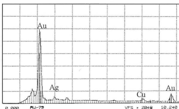
Abb. 7: EDX-Spektrum eines besonders silberarmen Metallpartikels. Der Silberpeak ist nur noch schwach zu erkennen, dafür treten Kupfer und einige andere Elemente (Silizium, Calcium, Eisen) aus dem Untergrund hinzu.
