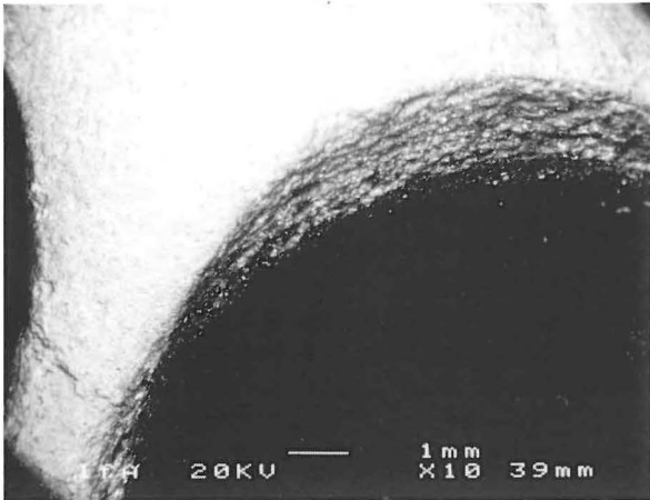
Abb. 3: RE-Bild der Innenwand einer Vertiefung der Form Z 1. Die hellen Punkte sind Metalltröpfchen, der Boden der Form erscheint schwarz. Auf der Oberfläche der Keramik überstrahlen Aufladungserscheinungen das Bild.
