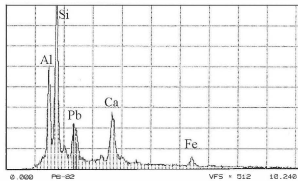
Abb. 8: EDX-Spektrum des verglasten Bodens einer Vertiefung. Neben den typischen Peaks der silikatischen Keramik fällt der deutliche Bleipeak (links, bei ca. 2,4 KeV) auf. Man beachte die gegenüber den vorigen Spektren um den Faktor vier veränderte Skalierung (VFS 512)!
