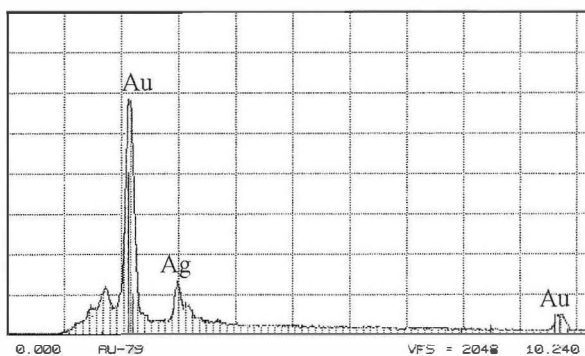
Abb. 6: EDX-Spektrum eines silberreichen Metallpartikels. Die Intensität des Silberpeaks ist deutlich geringer als in Abb. 5, der Gehalt an Silber entsprechend geringer.
